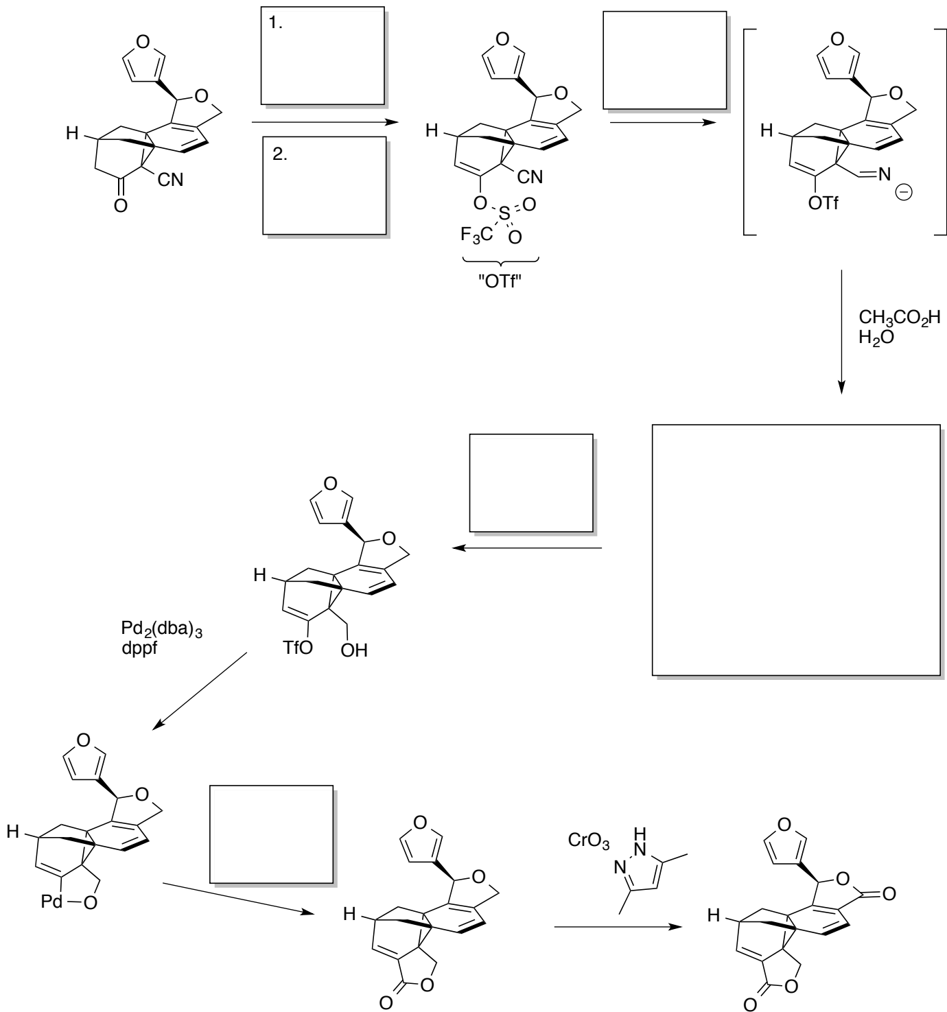
(+)-salvileucalin B
